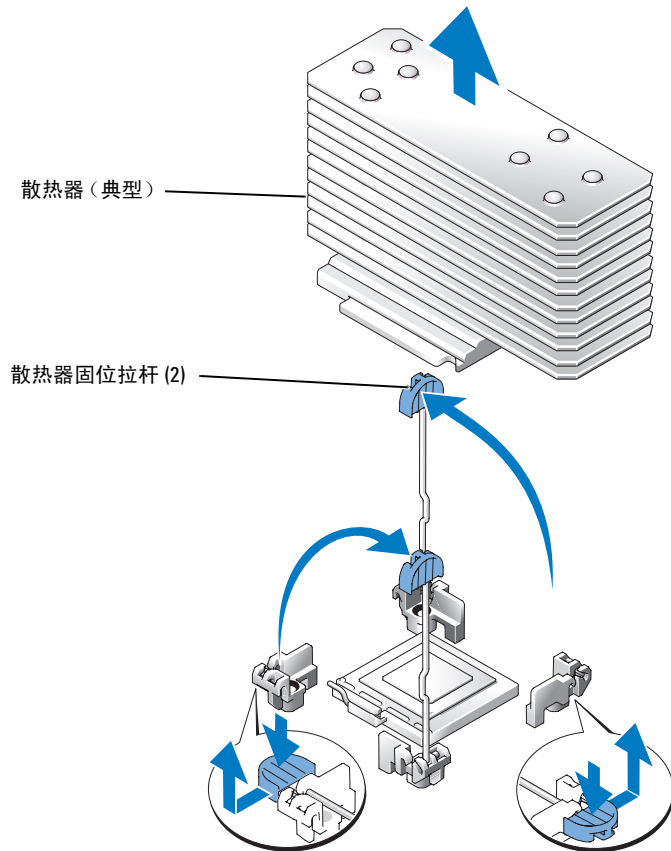
图 1-1. 装卸散热器
